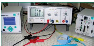
Prüfung DIGIFORCE® 9310
