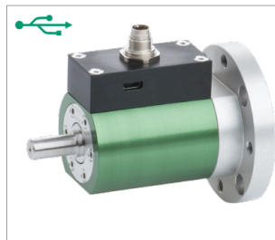
8625 mit Flansch
