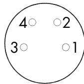
Stecker Vorderansicht M8 IEC
