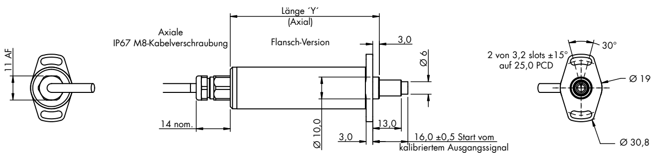
Maßzeichnung 2 – Schubstange mit Gewinde; Axiale Kabelverschraubung
