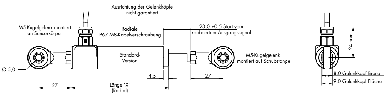
Maßzeichnung 3 – Schubstange und Gehäuse mit Kugelgelenkkopf; Radiale Kabelverschraubung
